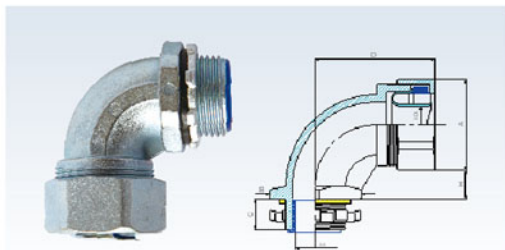
TYPE ZGLM (外螺紋接頭90°)
